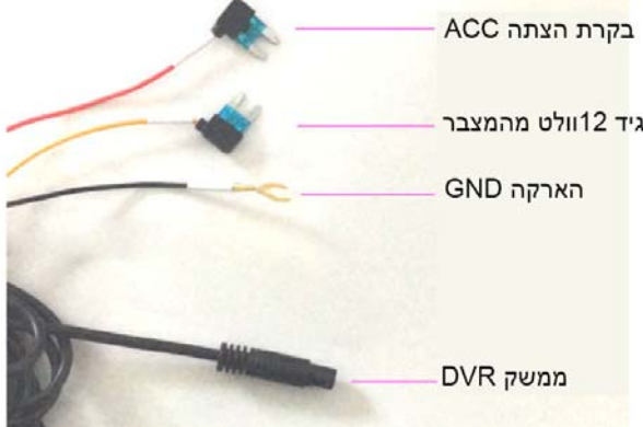
איור 1 – תרשים חיווט
